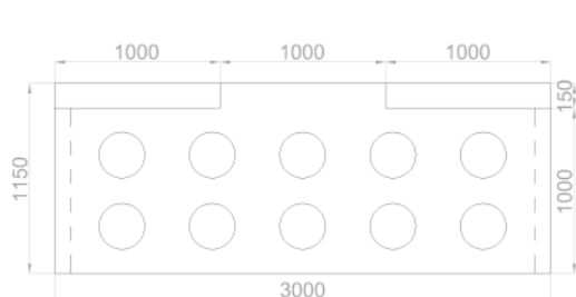
Treeblock - vooraanzicht
