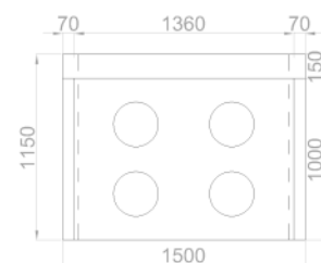
Treeblock - zijaanzicht
